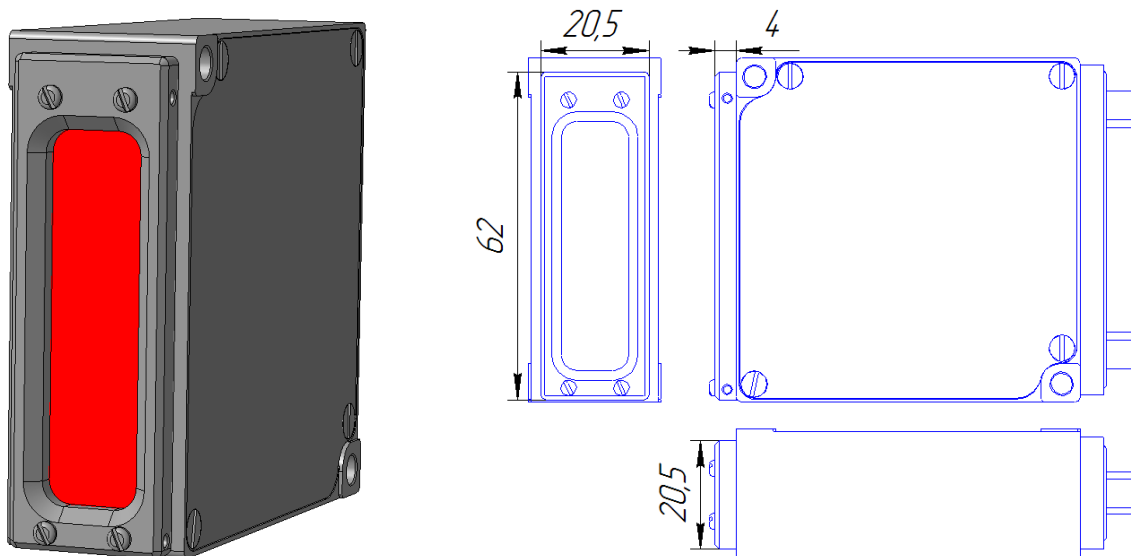
Датчик со сменным защитным стеклом
