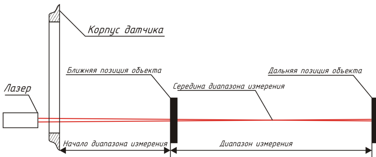
Рис 1. Схема позиции объекта измерения
