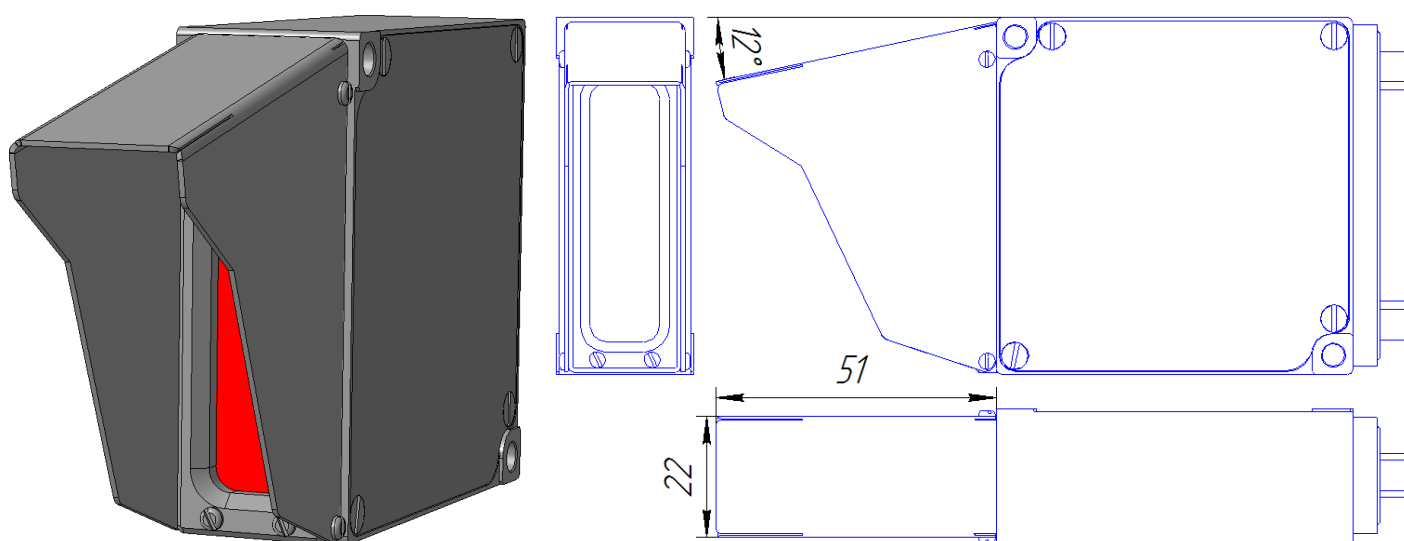
Датчик с защитной блендой (*сменным защитным стеклом)
