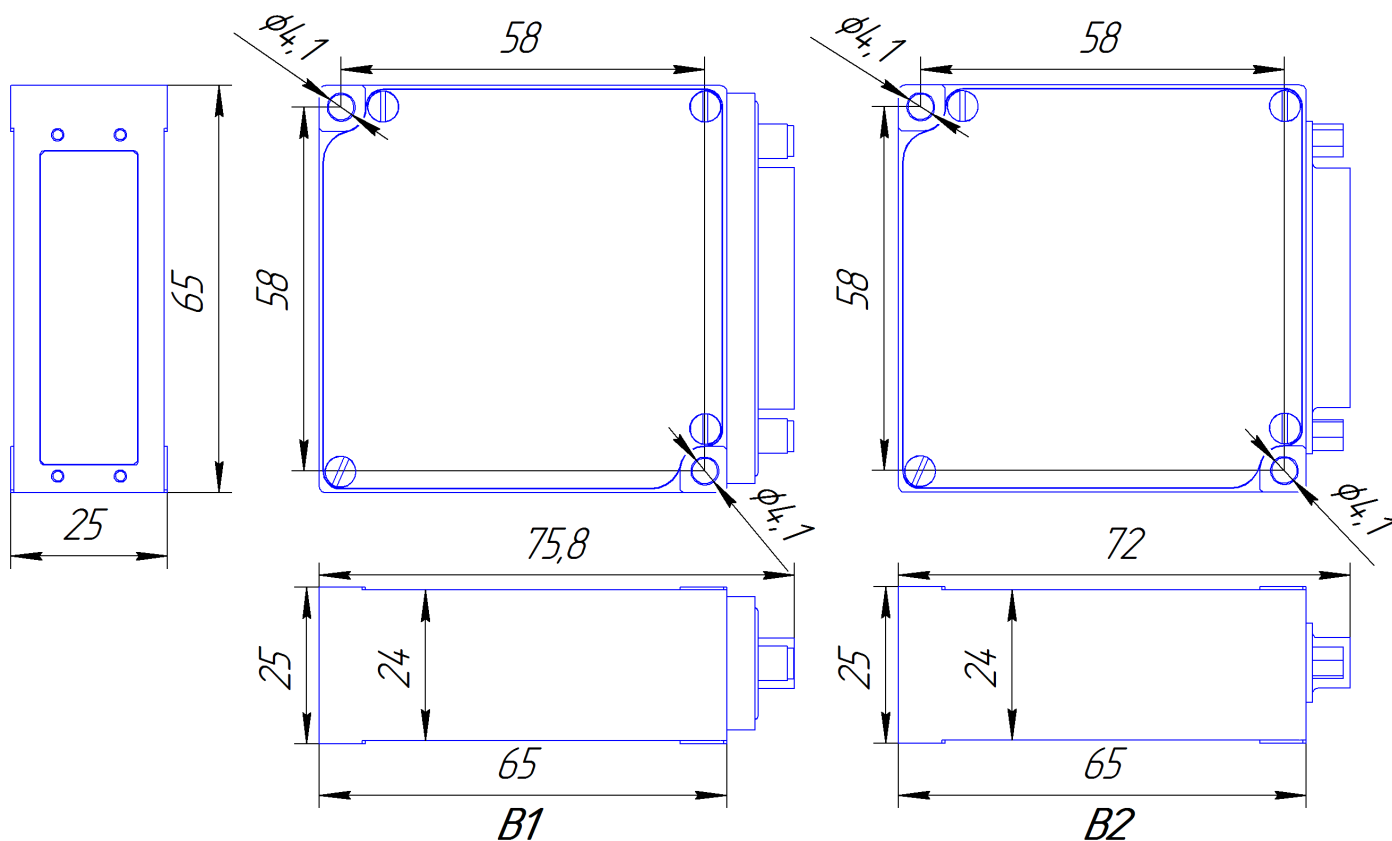
Рис 2. Габаритные размеры датчика с разъемом D-SUB25. B1 - корпус IP67; B2 - корпус IP60;
