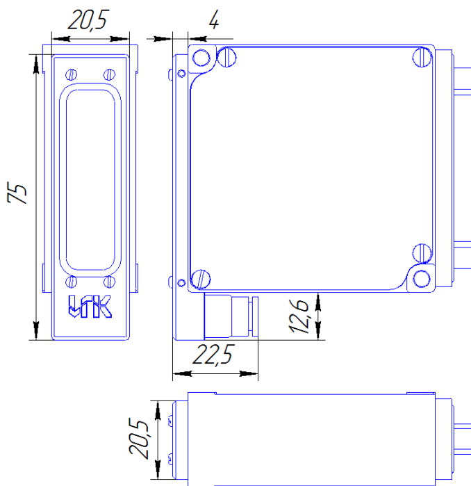
Датчик с опцией обдува сжатым воздухом (*сменным защитным стеклом)
