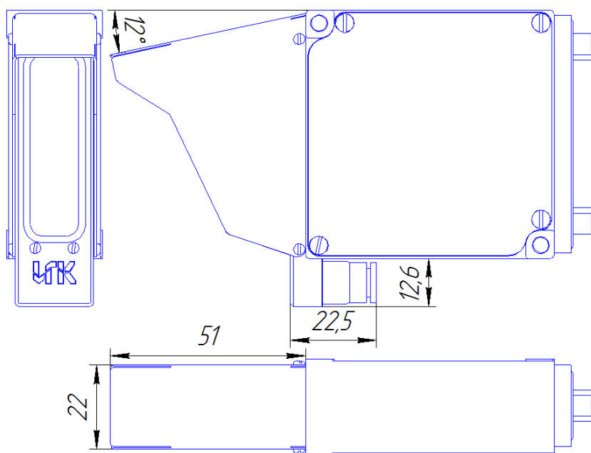
Датчик с опцией обдува сжатым воздухом и защитной блендой (*сменным защитным стеклом)
