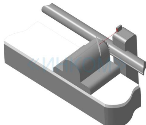
Следящая система управления, датчик управляет перемещением поддерживающего люнета фрезы
